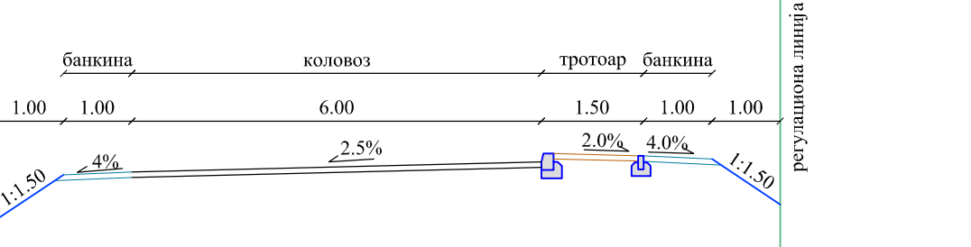
ПРЕСЕК 2-2
