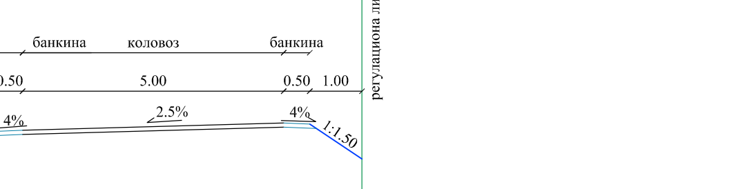
ПРЕСЕК 4-4
