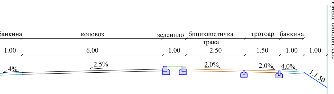
ПРЕСЕК 1-1
