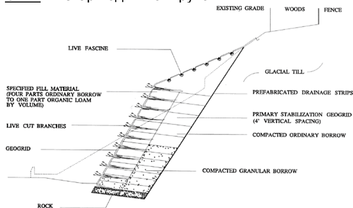
Сл. 1-Плетари од живог прућа
