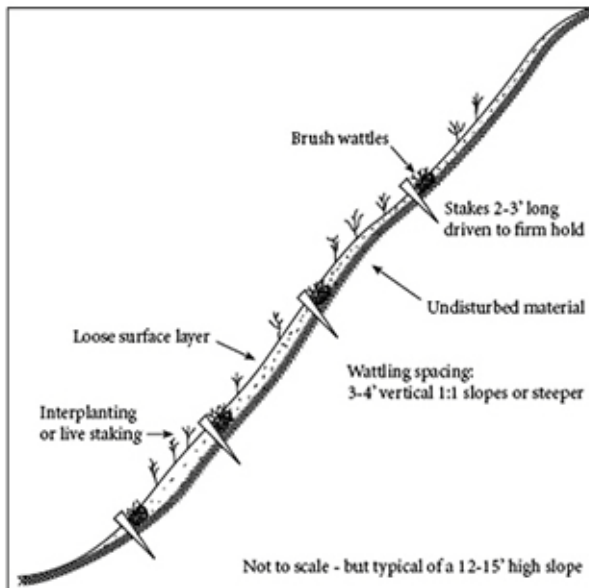
Сл. 3- Комбинација кочића и жбунастих врста
