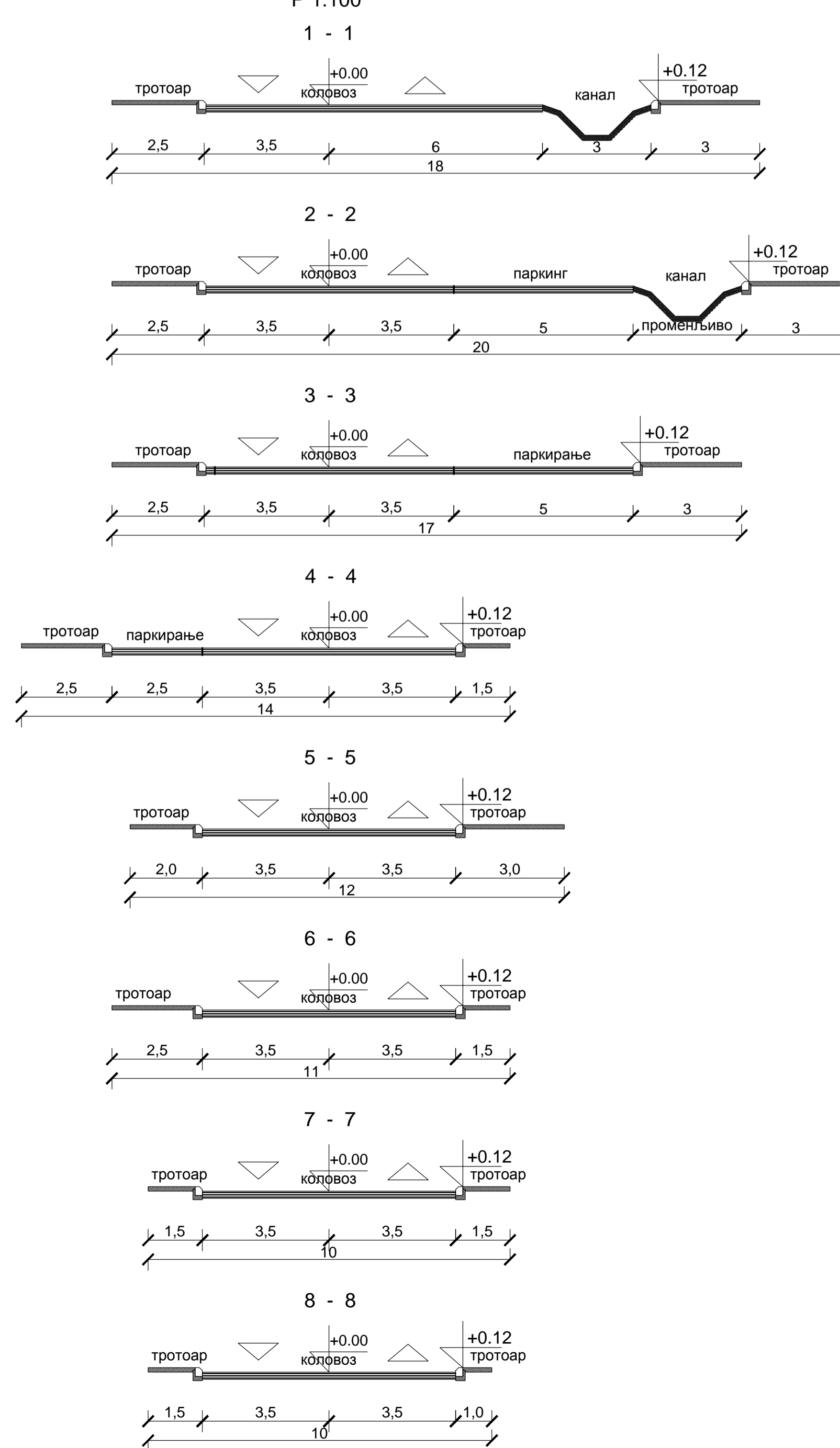
ТИПСКИ ПОПРЕЧНИ ПРОФИЛИ ПУТА Р 1:100
