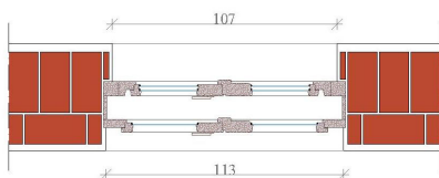
ПРЕСЕК 1-1 Р 1:20
