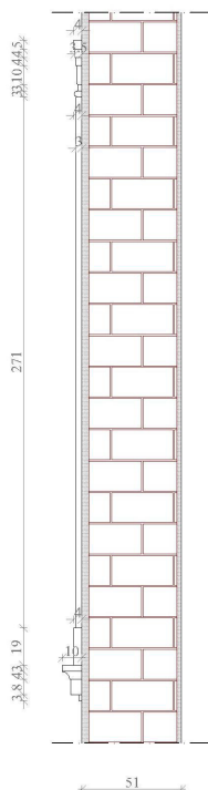
ПРЕСЕК 1-1 Р 1:20
