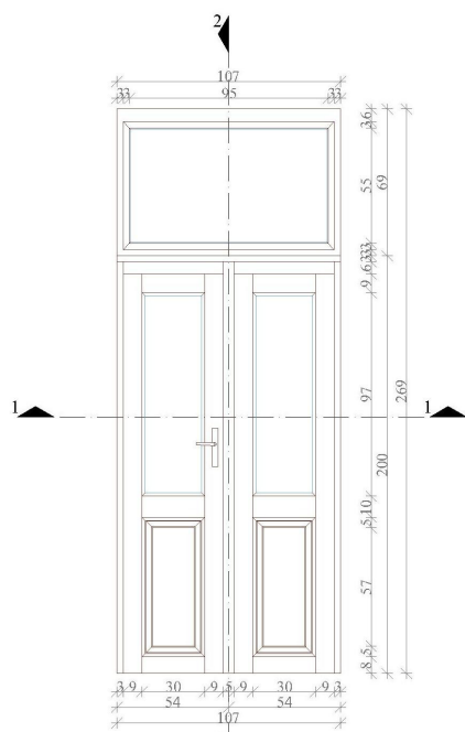
ИЗГЛЕД Р 1:20
