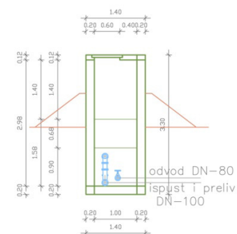
PRESEK B-B POSTOJEĆE KAPTAŽE SA IZVORIŠTEM
