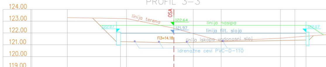
PROFIL 3-3
